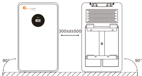
Podłozie (instalacja w dwóch rzędach)
