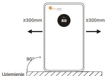
Podłozie (instalacja w dwóch rzędach)
