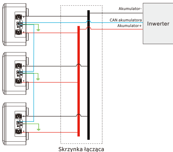
Rysunek 4-1 Połączenie równolegle trzech zestawów akumulatorów
