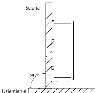
Podłozie (instalacja w dwóch rzędach)
