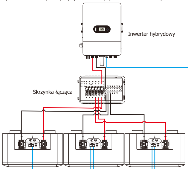
Rysunek 4-1 Połączenie równolegle trzech zestawów akumulatorów
