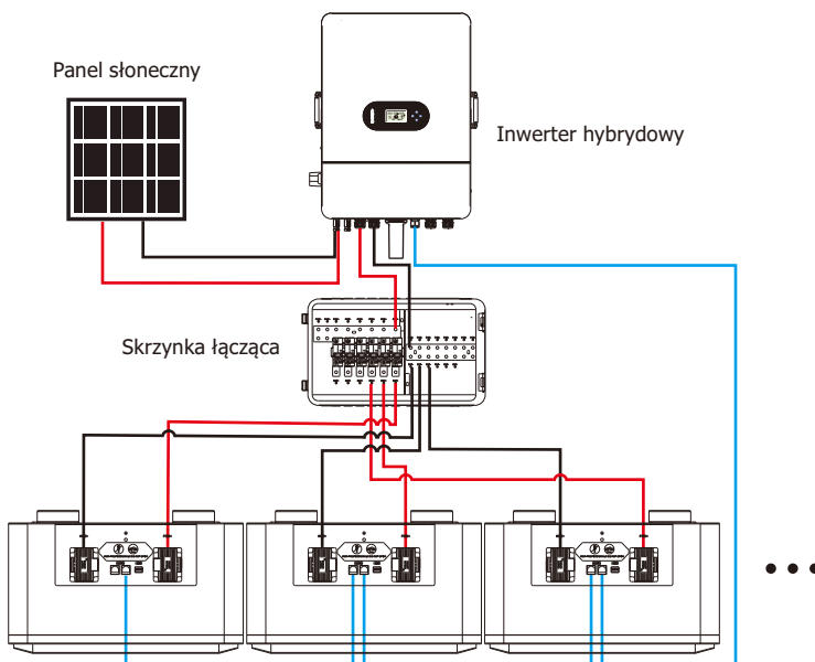
Rysunek 3-2 Schemat połączenia wielu akumulatorów w układzie równoległym
